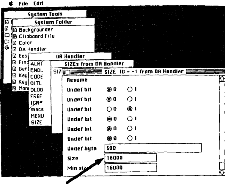
شكل (٣-٩) : استخدام ResEdit في زيادة موقع ذاكرة مساعد المكتب Handler .
